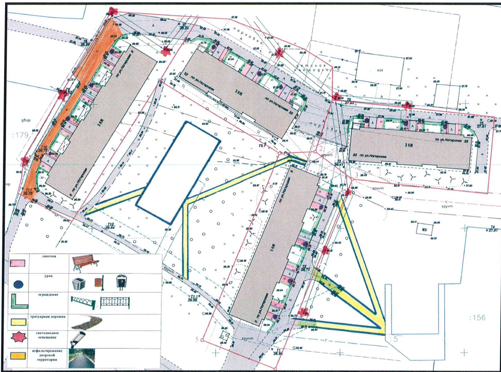
Схема планировочной организации земельного участка
